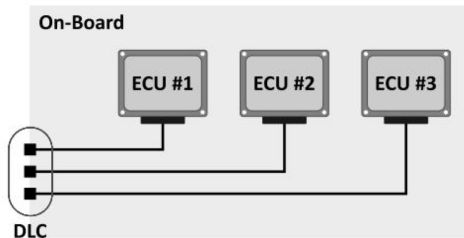
Abbildung 2.10: Punkt-zu-Punkt Verbindung für K-Leitung und SAE J1850.
