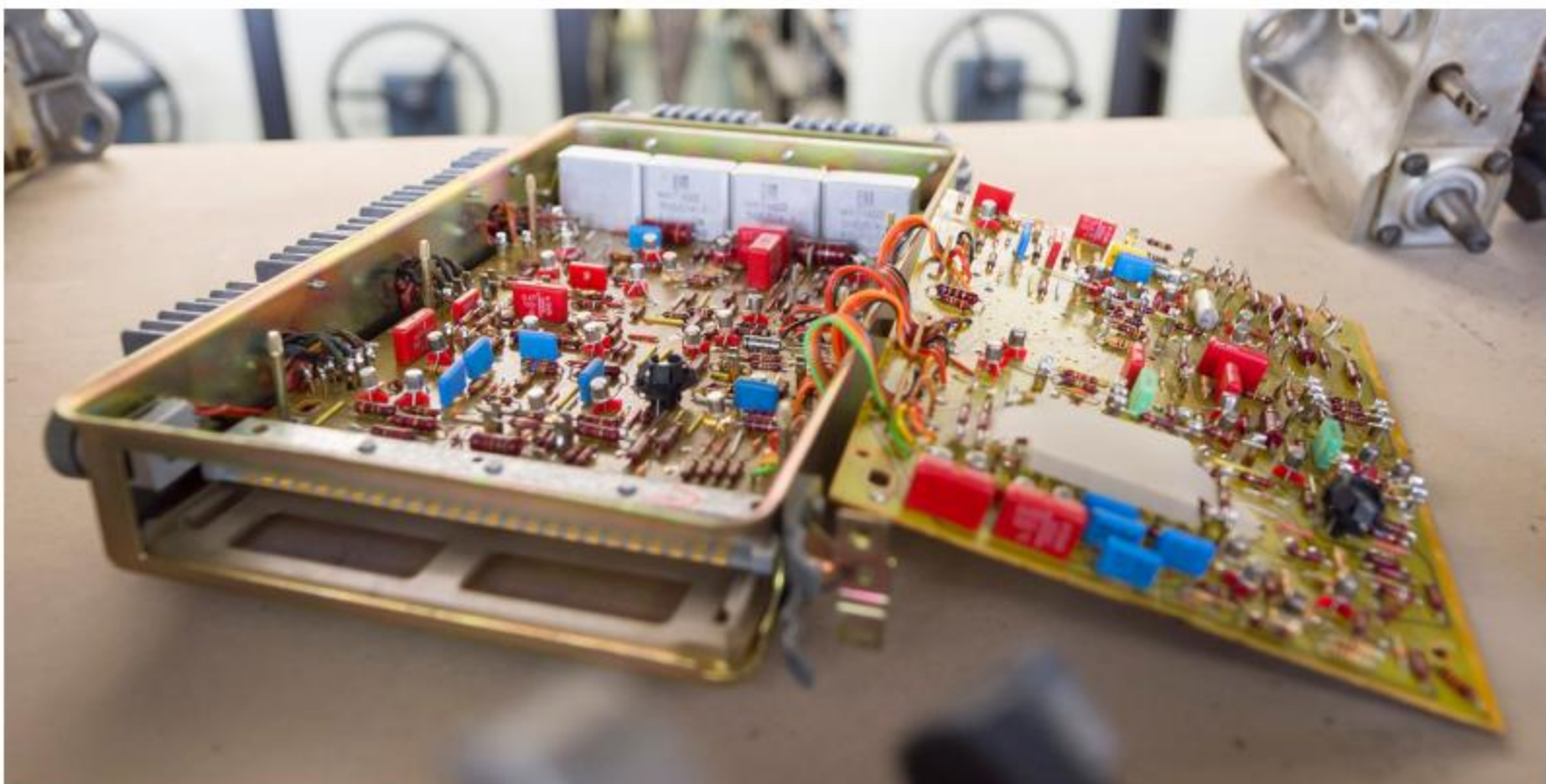
Abbildung 2.1: Die Jetronic bestand noch ausschließlich aus diskreten Bauteilen wie Widerstände, Kondensatoren, Transistoren etc. (Foto: Bosch).
